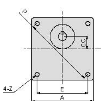
尺寸表 (mm)
