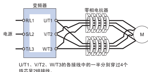
接线图c
