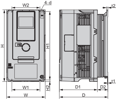
外形图 1
