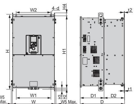
外形图 5
