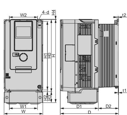
外形图 1
