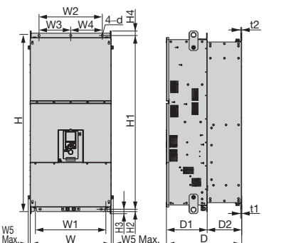
外形图 6
