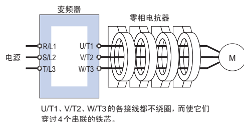
接线图b
