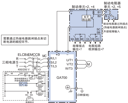
接线图C
