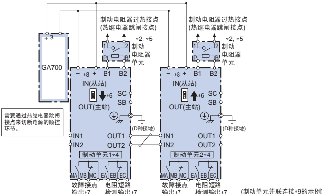
接线图D
