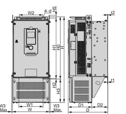
外形图 3
