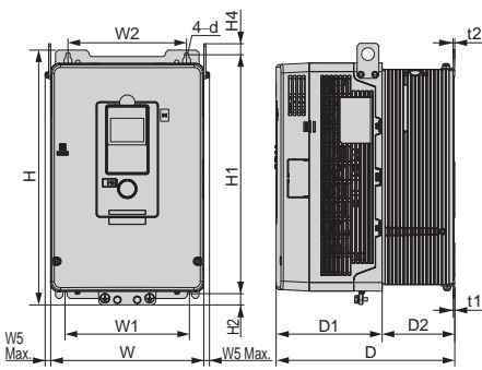
外形图 2
