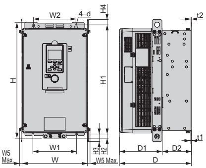
外形图 3
