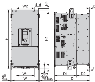
外形图 4
