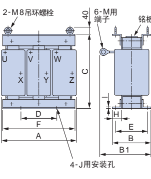
外形图2
