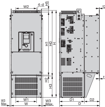
外形图 4
