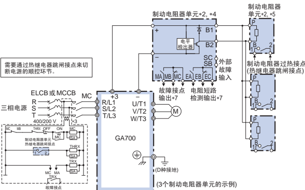
接线图E
