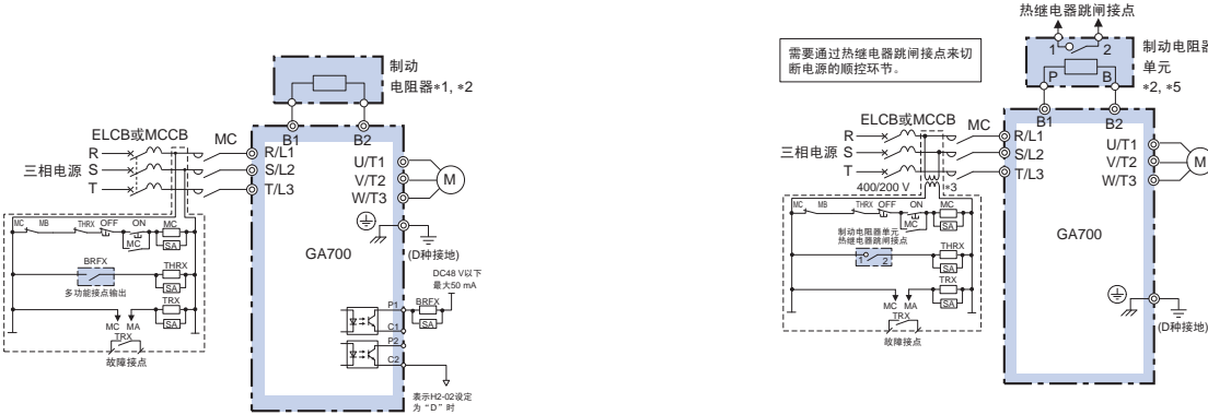
接线图A
