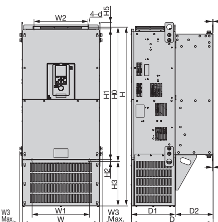
外形图 5
