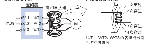
接线图a
