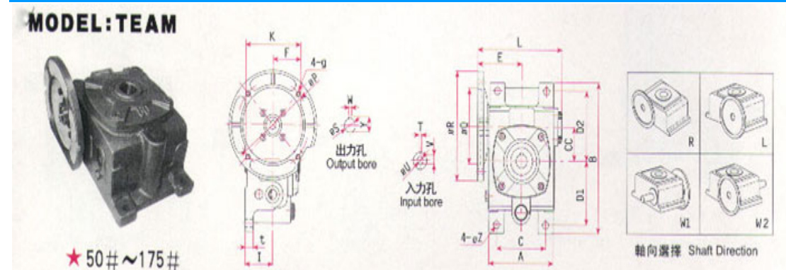
尺寸表 Dimension
