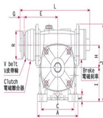
電磁剎車/離合器定格電壓DC 24V
