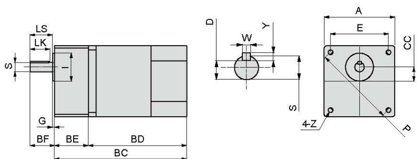
尺寸表 (mm)
