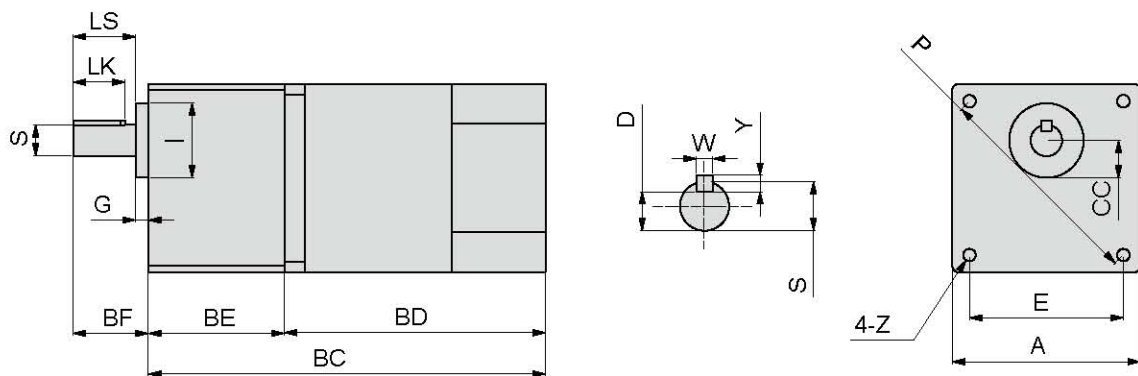
尺寸表 (mm)
