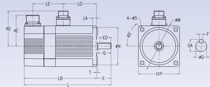
馬達外型圖
